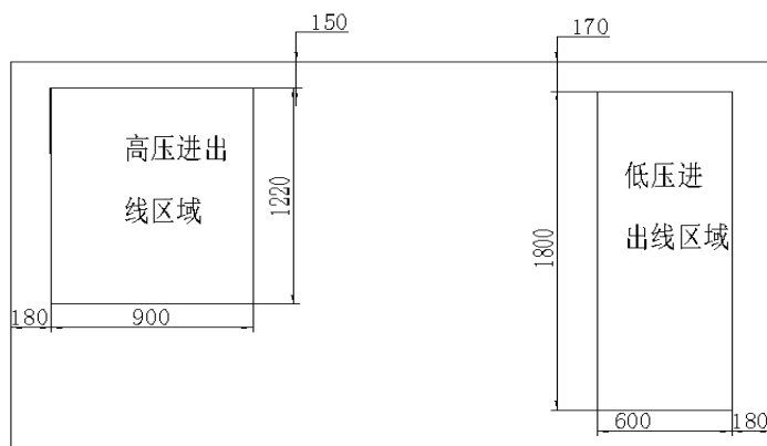
图 5 标准型高低压电缆孔布置图
